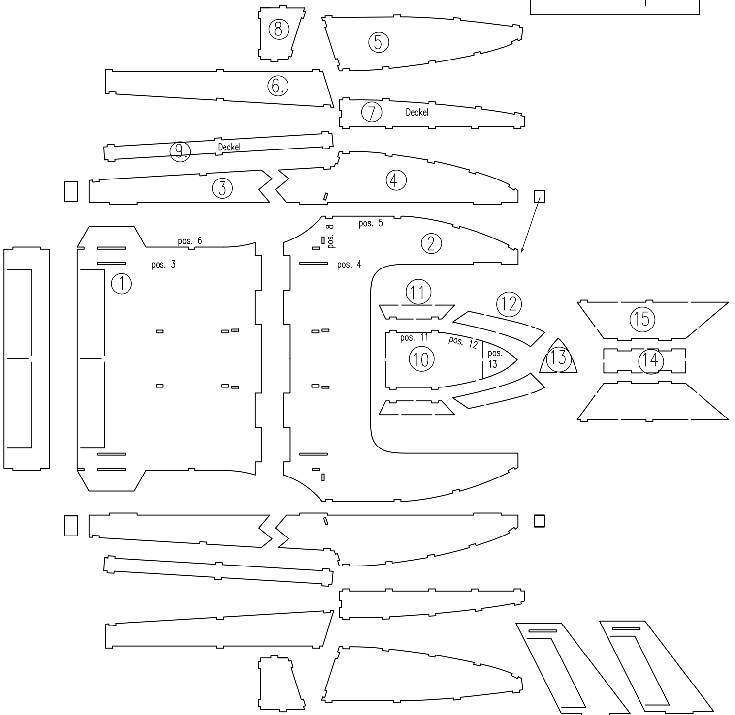
Flugboot Positionsplan
